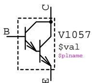
TR_BDT65 V?????
