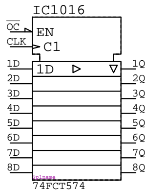
74FCT574
