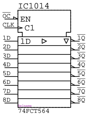
74FCT564
