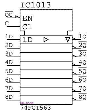
74FCT563
